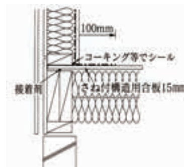
(d) コーキングでシールし、外壁の防湿フィルムを床合板に折り返す場合
