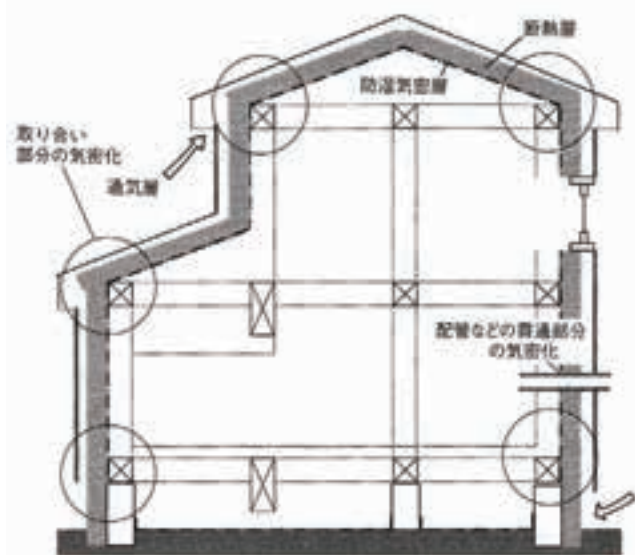
図 5.3.1 外張断熱工法
