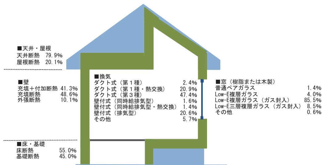
図 2.1.4 北海道の住宅の断熱仕様
