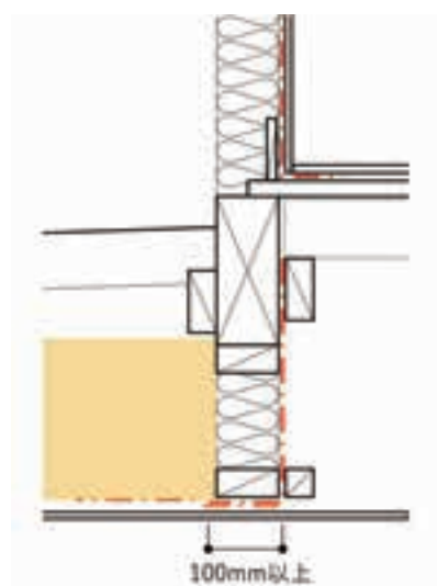
図 5.2.13 下屋部分の先張り防湿フィルムの施工例
