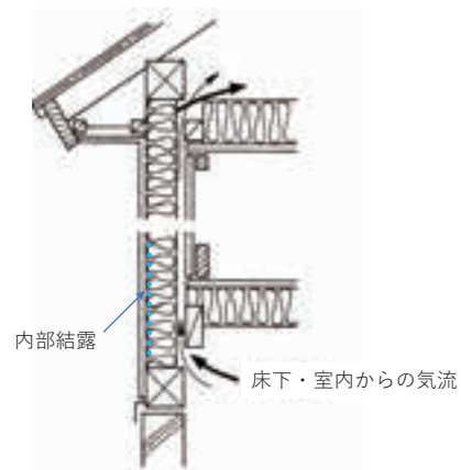
図 2.1.3 気密層の欠損が引き起こす問題
