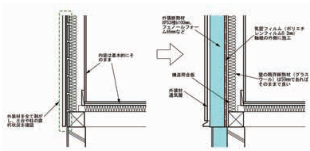
図 8.2.16 外壁と1階床の取合い部
