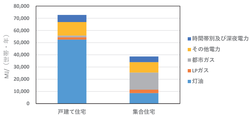
図 2.1.14 北海道の戸建て住宅と集合住宅のエネルギー消費量 出典：北海道消費者協会「平成 30 年度北海道家庭用エネルギー消費実態調査報告書」
