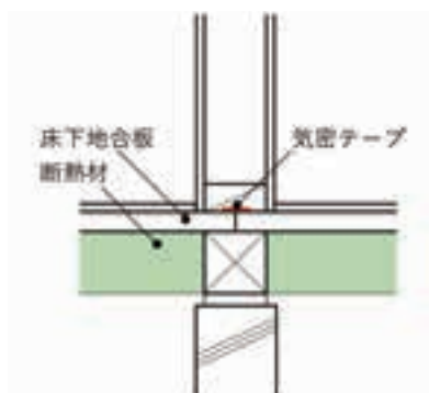
図 5.2.6 最下階床と間仕切壁の取合い部
