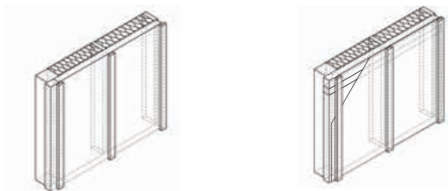
図 5.1.7 外壁の断熱上の問題点と対策
