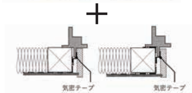
(b) サッシの内側からシールする場合
