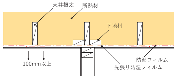
図 5.4.4 屋根直下の天井と内部壁枠組の取合い部
