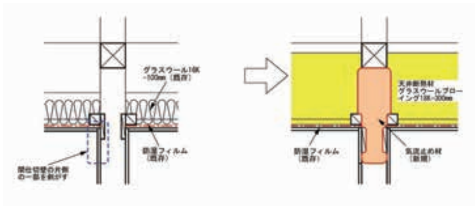
図 8.2.7 間仕切壁と最上階天井の取合い部（床断熱、基礎断熱工法の場合）
