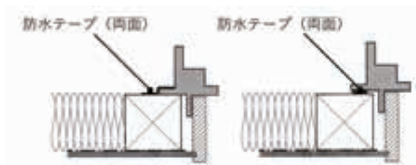
(a) サッシの外側からシールする場合
