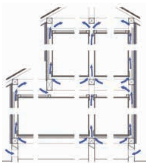
図 8.2.1 壁内気流の生じている住宅の断面
