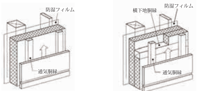
(a) 断熱材を1層張りとした場合
