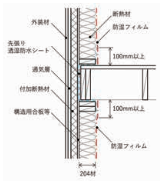
図 5.4.2 中間階床と外壁の取合い部
