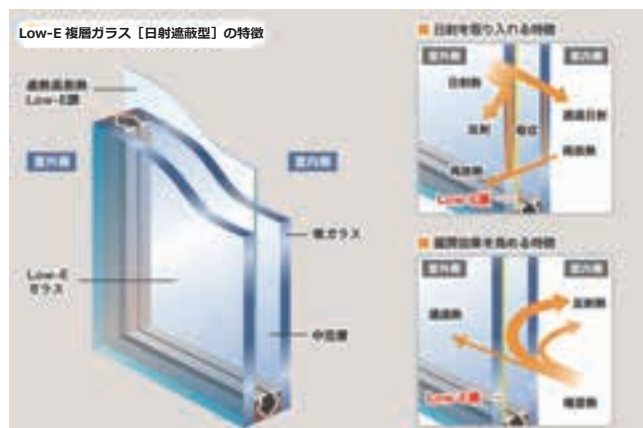
図 3.3.4 Low-E 複層ガラス【日射遮蔽型】
