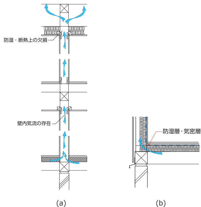
図 3.2.17 気流止めを施工しない場合に起こる壁内気流の例
