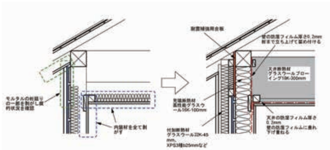
図 8.2.12 外壁と桁の取合い部
