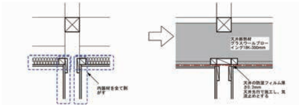
図 8.2.14 間仕切壁と最上階天井の取合い部
