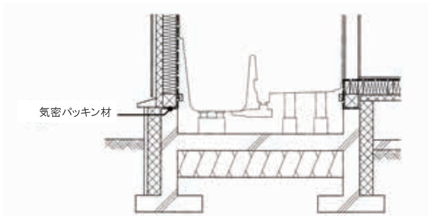
図 5.1.4 ユニットバス下部の断熱施工例
