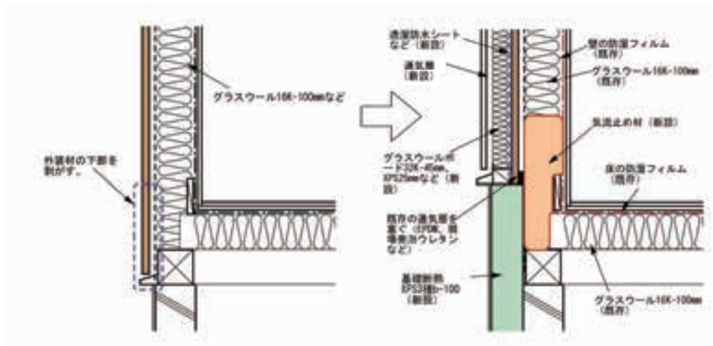
図 8.2.3 外壁と1階床の取合い部
