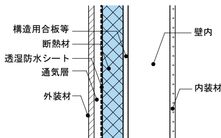
図 3.2.4 外張断熱工法・発泡プラスチック系断熱材を使用した例
