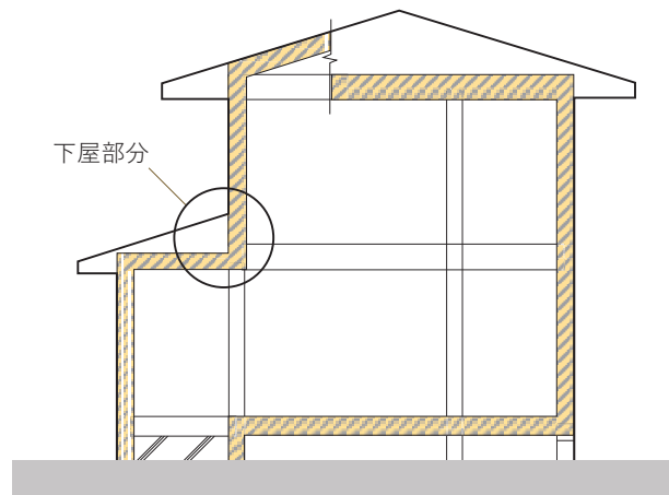
図 5.2.12 工程5 下屋部分の天井および下がり壁の施工
