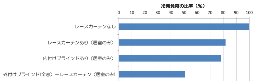
図 2.2.3 日射遮蔽部材による冷房負荷
