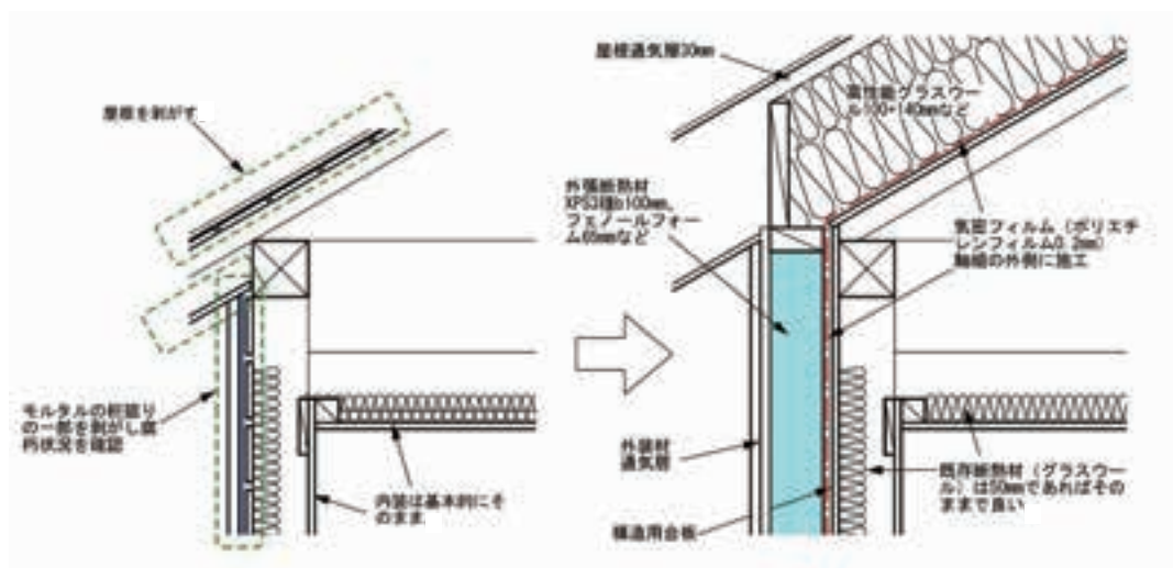
図 8.2.18 外壁と桁の取合い部
