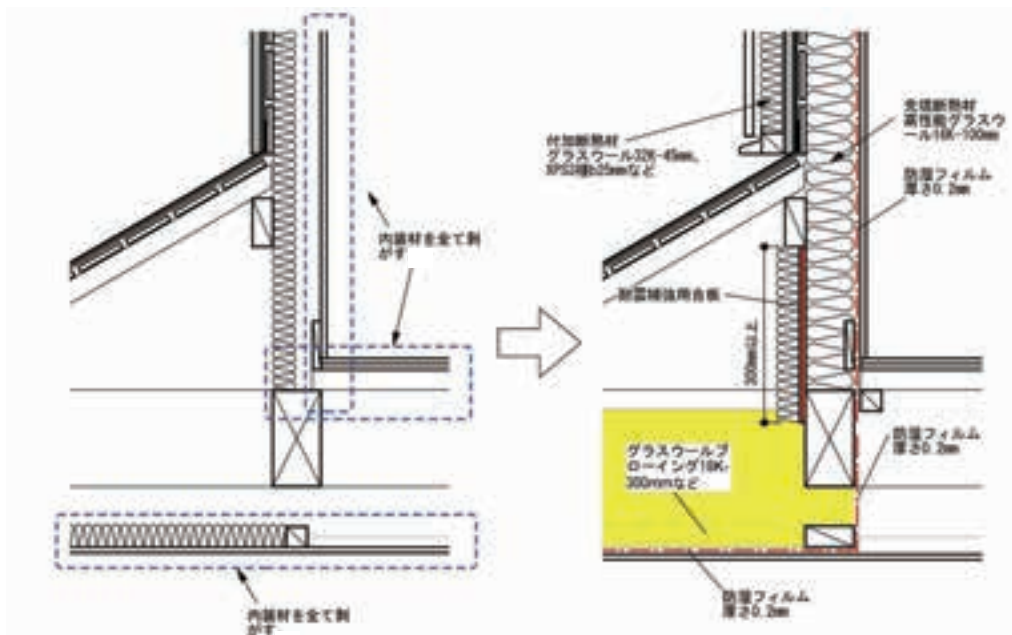
図 8.2.15 下屋部分
