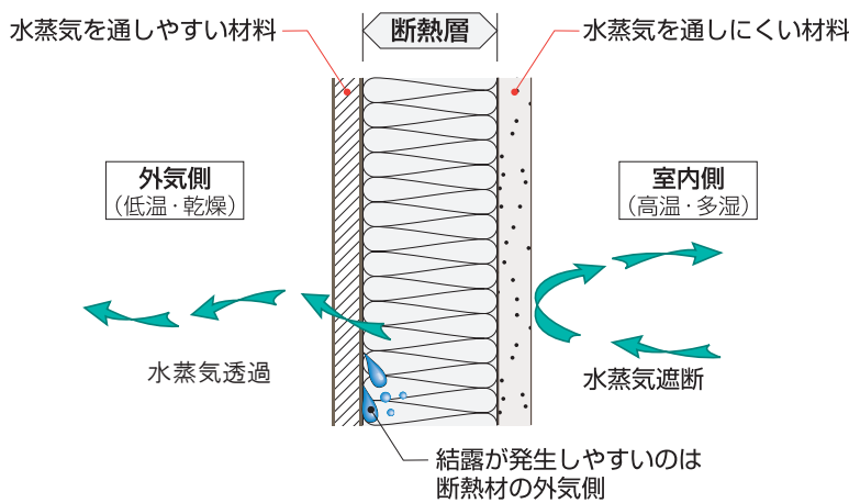
図 3.2.2 壁体内の水蒸気の流れ
