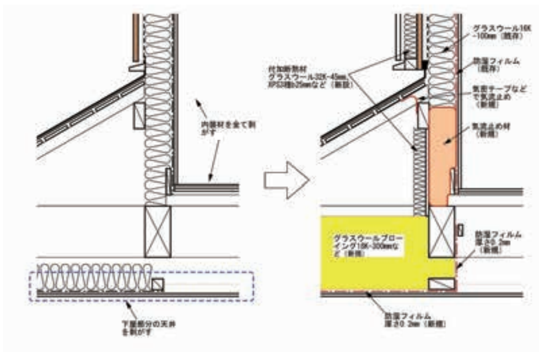
図 8.2.8 下屋部（床断熱、基礎断熱）
