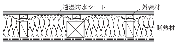
図 3 2.16 不適切な施工例
