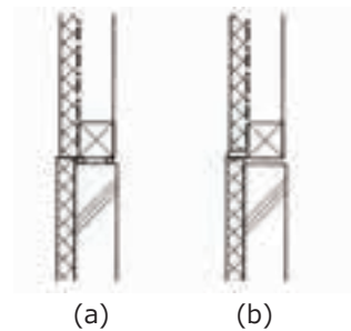
(a) 基礎上端部に気密パッキン材を施工 (b) 断熱材の継目に現場発泡断熱材を施工
