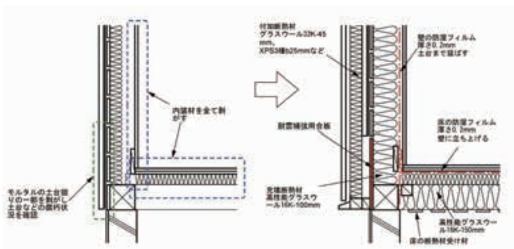
図 8.2.9 外壁と1階床の取合い部
