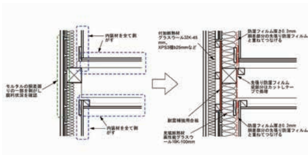
図 8.2.11 外壁と胴差の取合い部
