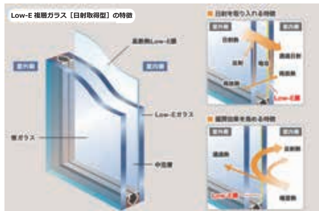
図 3.3.3 Low-E 複層ガラス【日射取得型】
