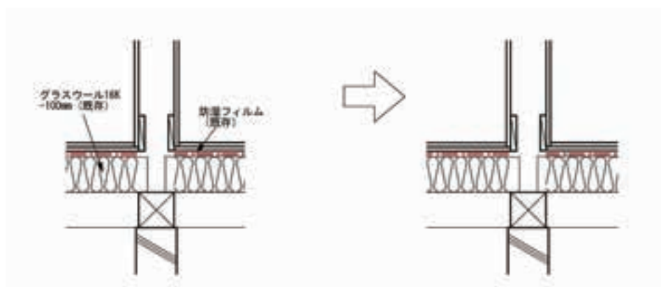
図 8.2.6 間仕切壁と１階床の取合い部（基礎断熱工法の場合）
