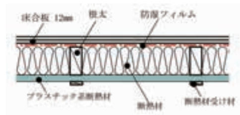
図 5.1.2 プラスチック系断熱材による付加断熱の例
