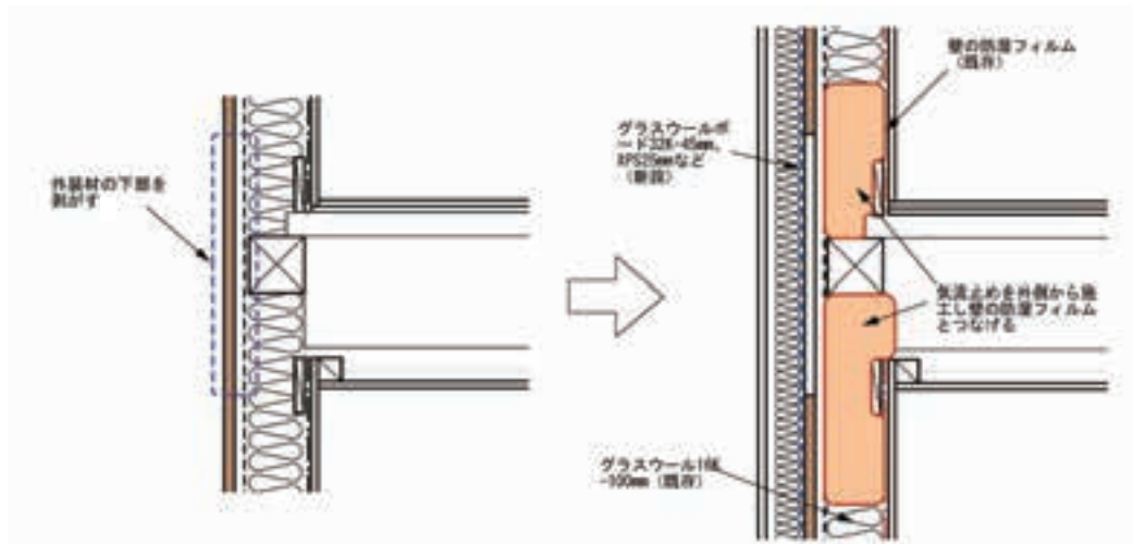
図 8.2.4 外壁と胴差の取合い部（床断熱、基礎断熱）
