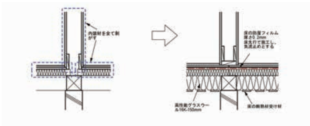
図 8.2.13 間仕切壁と1階床の取合い部
