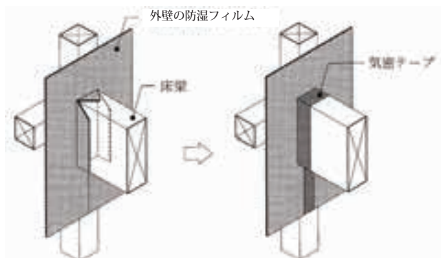
図 5.5.2 梁が防湿フィルムを貫通する部分の施工例
