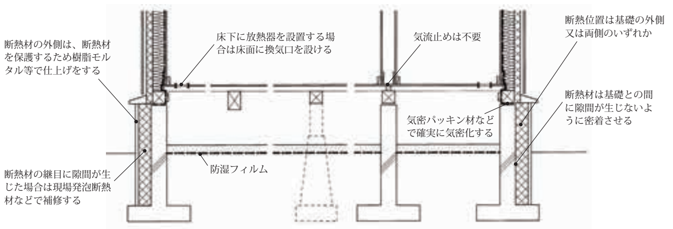
図 5.1.6 基礎断熱の例
