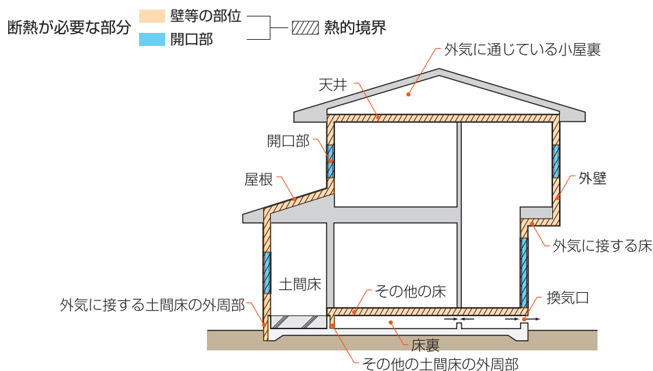
図 3.2.1 熱的境界
