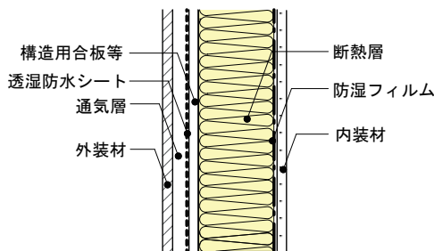
図 3.2.3 充填断熱工法・繊維系断熱材を使用した例
