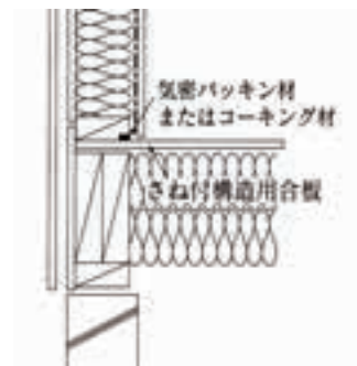
(b) 下枠に気密パッキン材を詰め込む場合
