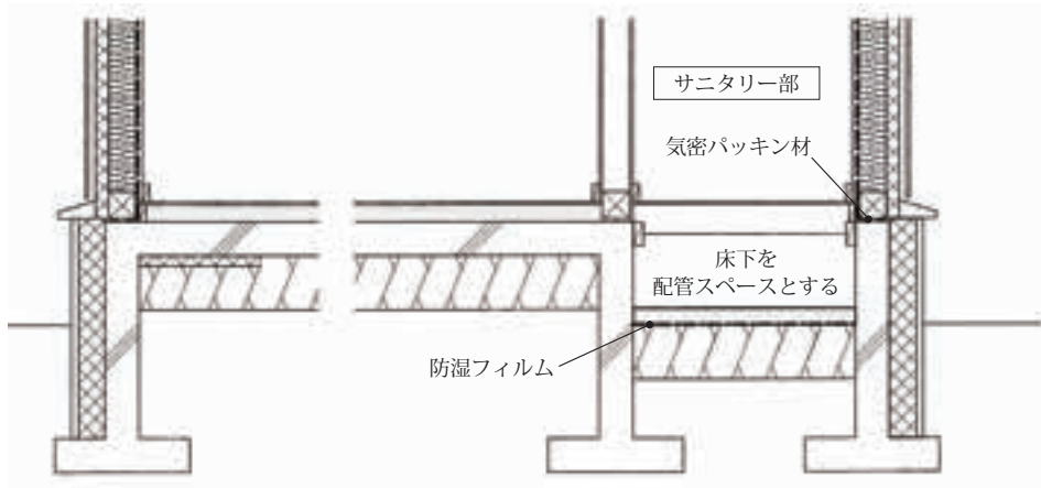
図 5.1.5 土間床の基礎断熱の例
