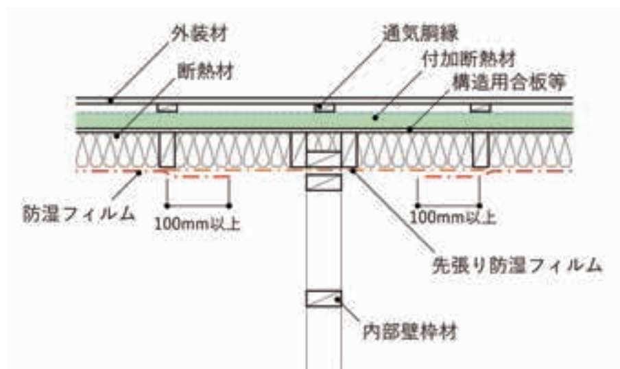
図 5.4.3 外壁と内部壁枠組（間仕切壁）の取合い部
