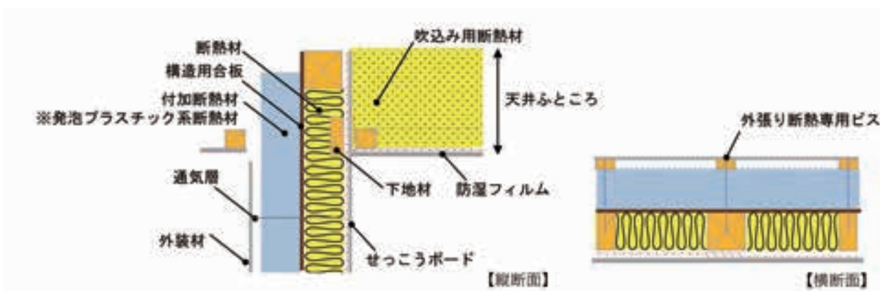
(a) 外張り断熱専用ビスを使用して柱・間柱に固定する方法 図7.1.1 付加断熱の厚さを増加した高断熱壁体の例
