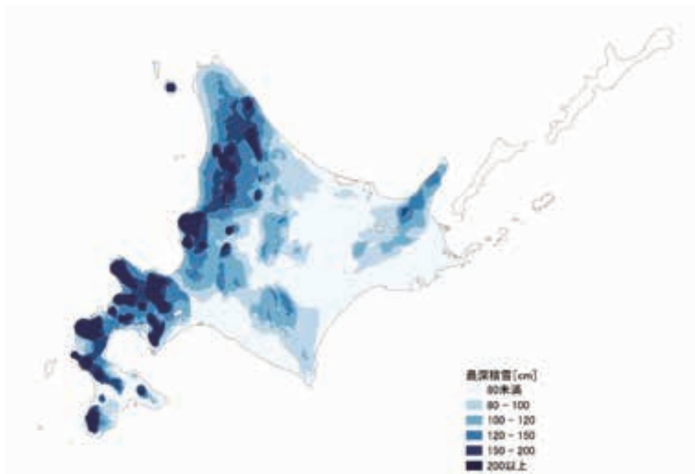
図 1.1.3 北海道の最深積雪の分布
