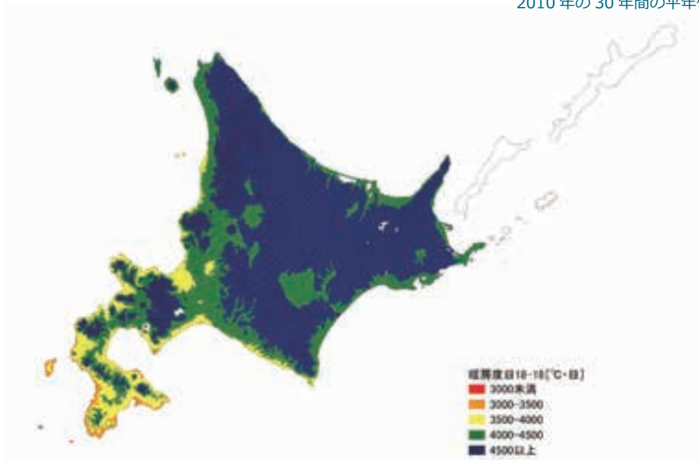
図 1.1.2 北海道の暖房度日の分布
