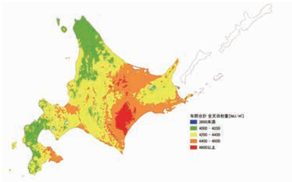
図 1.1.4 北海道の年間日射量の分布
