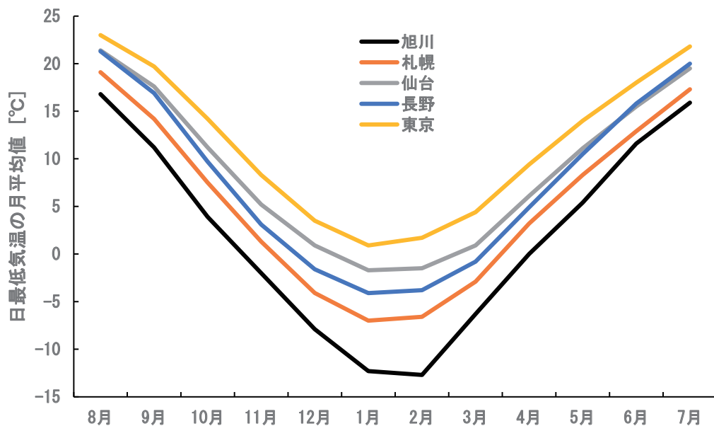
気象庁のデータによる。1981-2010年の平年値 図 1.1.1 北海道と本州各都市の月別の日最低気温の平均値
