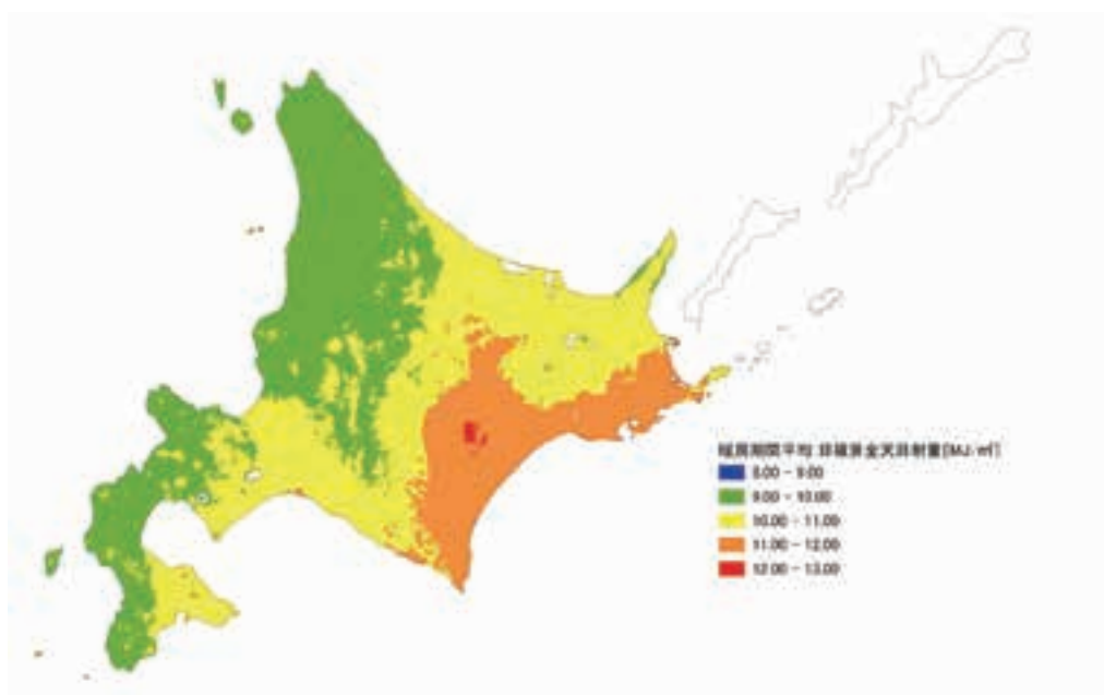
図 1.1.5 北海道の暖房期日射量の分布
