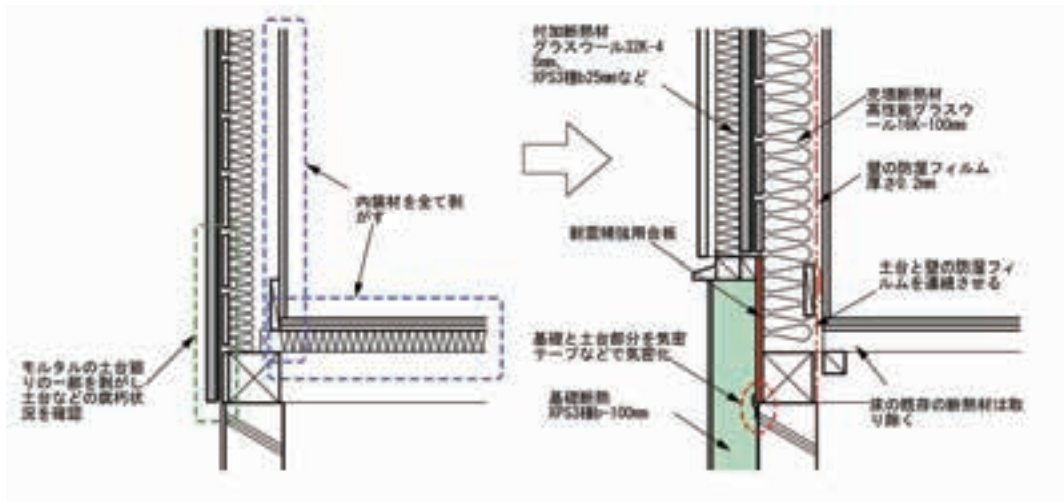
図 8.2.10 外壁と1階床の取合い部（基礎断熱工法）
