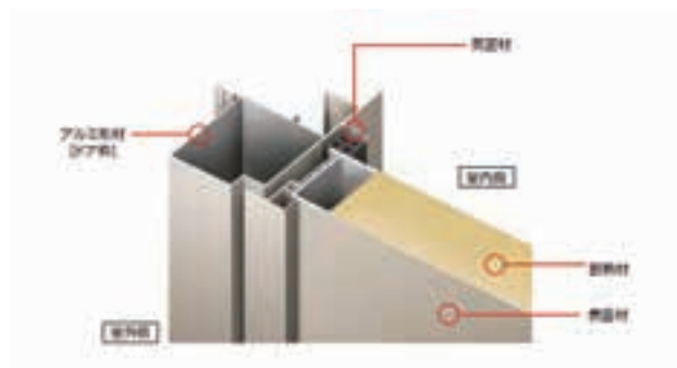
図 3.3.9 フラッシュドアの構造
