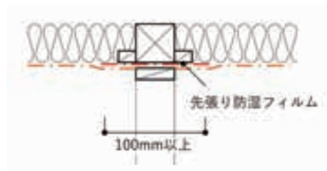
図 5.2.9 外壁と間仕切壁の取合い部
